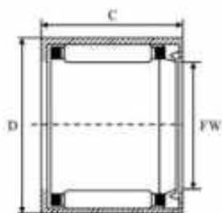
HK..RS
