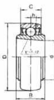
UK2
