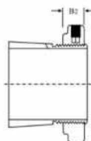
HA..E, HE..E
