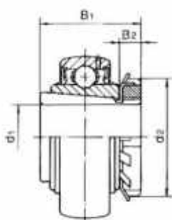
UK2+H
