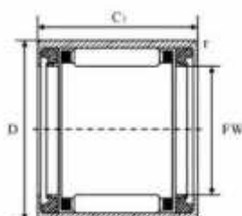
HK..IRS
