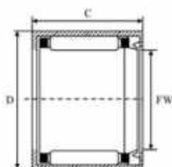
HK..RS
