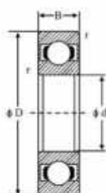
2RS
