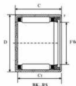
BK..RS
